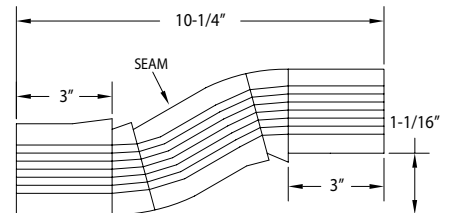
ABO2A34A A-Offset
