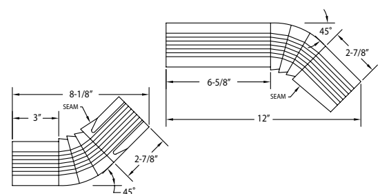
ABO2A34A A-Offset
