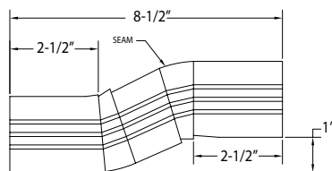
ABO1123A A-Offset
