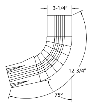
ABE245 B-Elbow
