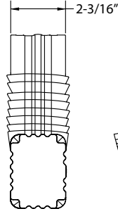
AAE245 A-Elbow
