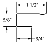
AJ58 - -
