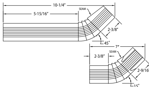
ABO2A23A A-Offset
