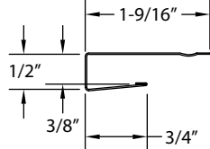
AWJ38 - -
