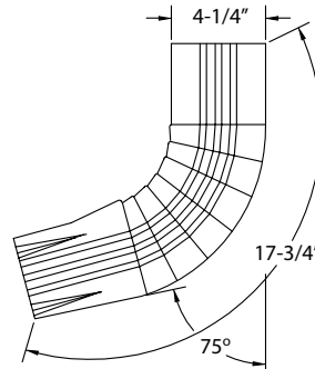
AAE245 A-Elbow
