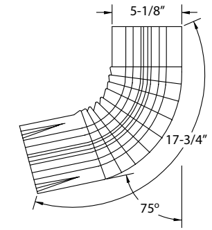
ABE245 B-Elbow
